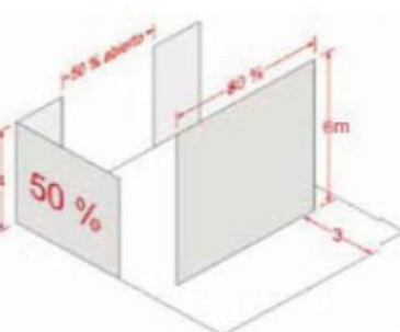
Cerramientos.
