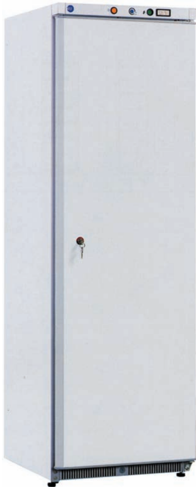
AN SALAMANCA Armario de refrigeración. 1 puerta ciega. Frio positivo. Cierre con llave Refrigerated cabinet. 1 blind door. Positive cold. Lock with key DIMENSIONES / SIZE 593 x 622 x 1874 mm CAPACIDAD / CAPACITY 343 L TEMPERATURA / TEMPERATURE 0° C a/to +8° C POTENCIA / POWER 175W/10A
