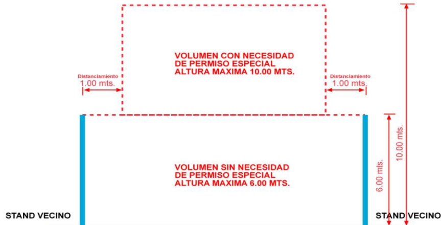
Esquema de elevación frontal
