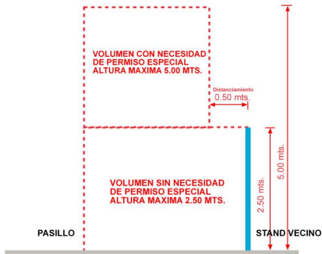
Esquema de elevación lateral
