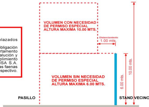
Esquema de elevación lateral
