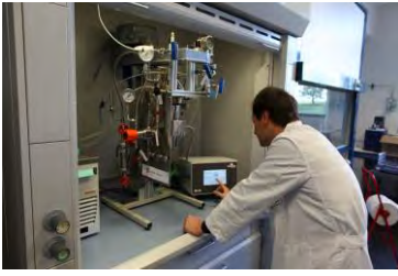
SEHICET. Sensor de detección de hidrógeno en los circuitos de centrales termosolares. CENER (Centro Nacional de Energías Renovables).
